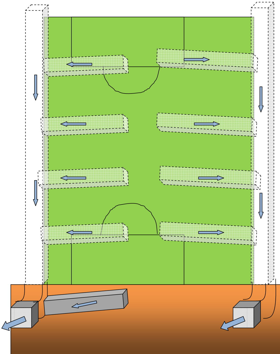
SISTEMA DI DRENAGGIO CAMPO DI CALCIO CON IDROSAC 500
