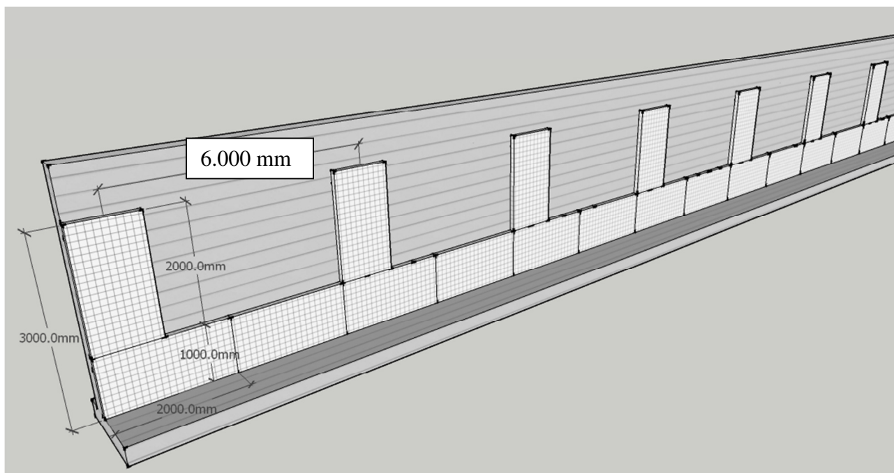
Fig.1. Disposizione a pilastri drenanti H=2, interasse di 6 m
